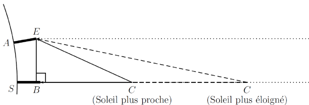
Figure 6 - Plus le Soleil C s'éloigne et plus l'angle C tend vers zéro et plus les droites passant par les points E et B tendent à devenir parallèles entre-elles
