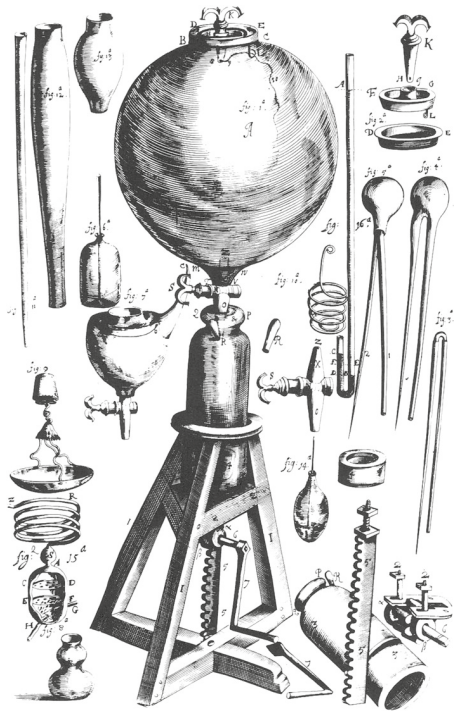
Document 12 - R. Boyle, Dessin de la pompe à air, extrait de Robert Boyle publié son ouvrage New experiments physico-mechanical touching the spring of the air , 1660.
