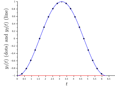
(d) Particle oscillations for \gamma = 0.2, T = 4\pi
