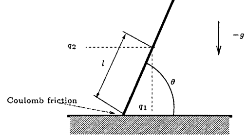
Fig. 2. Painlevé system.
