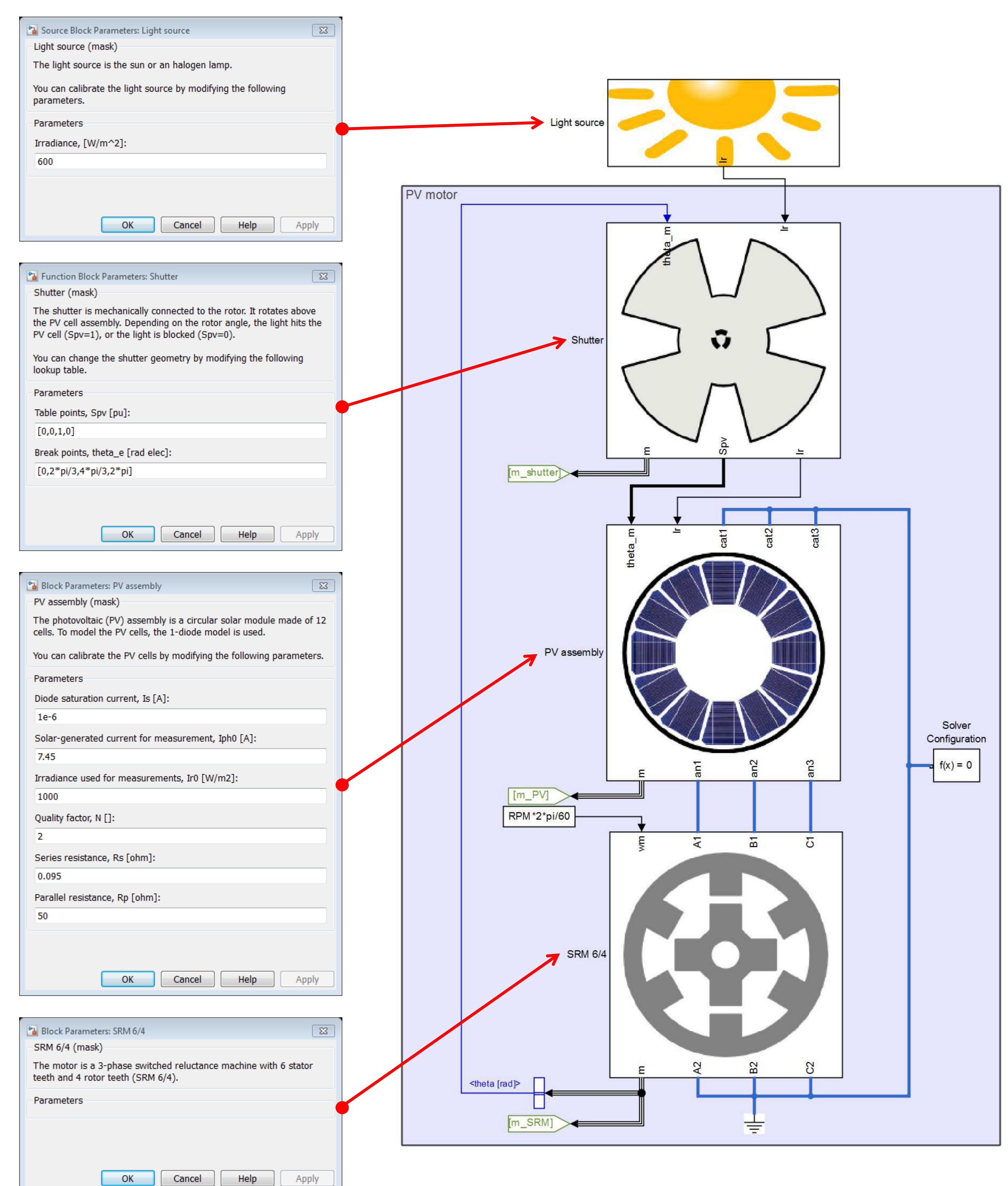
Fig. 3 - Modèle MATLAB/Simulink du moteur photovoltaïque.
