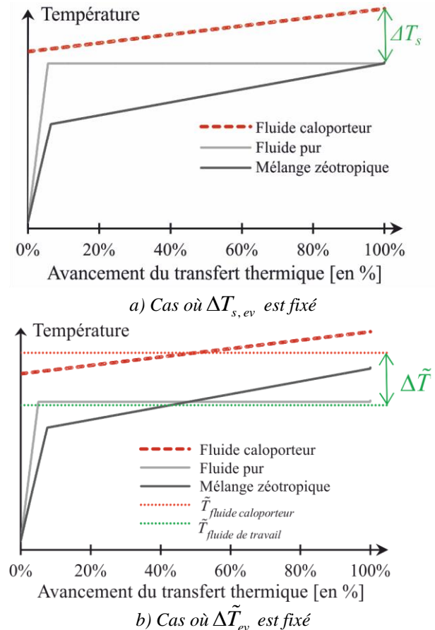
Figure 2 : Profils types d'évolution des températures dans un évaporateur au cours de l'avancement du transfert thermique
