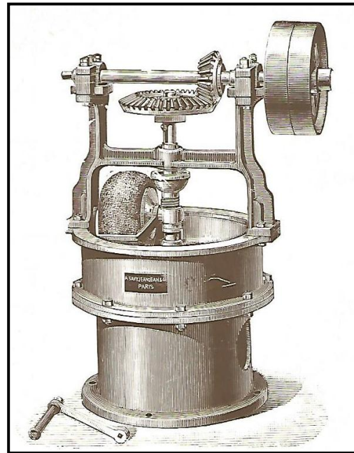
Mélangeur-broyeur
