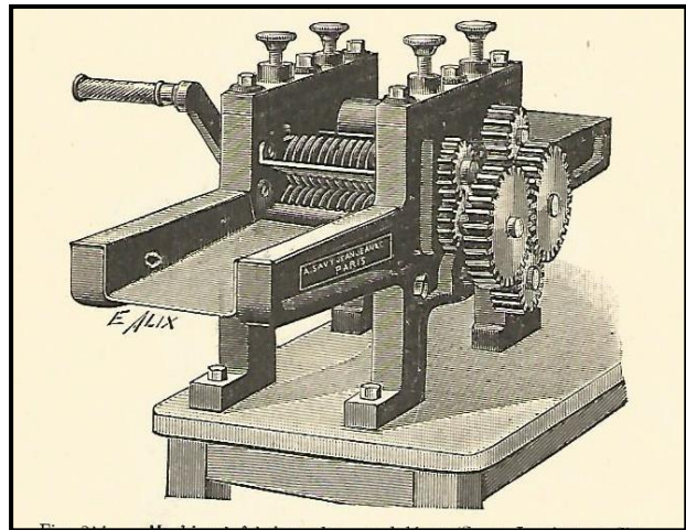
Machine à faire les magdaléons (pilules)
