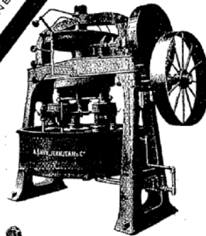
Conche circulaire
