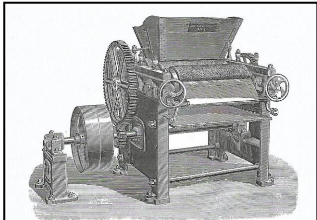
Broyeuse à trois cylindres en granit
