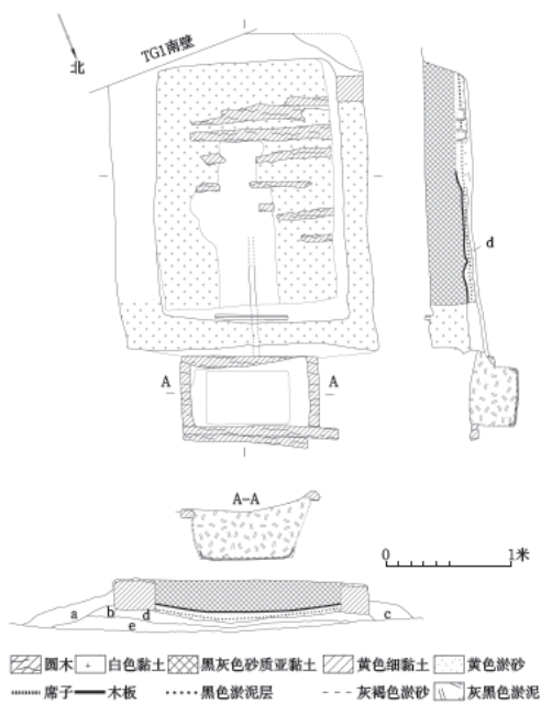
图五 YJ1平、剖面图
