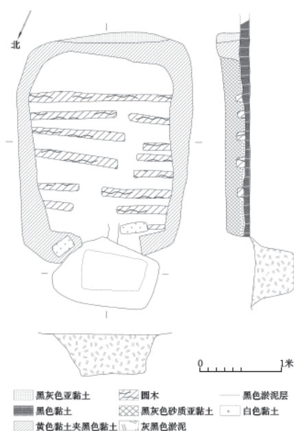
图七 YJ3平、剖面图
