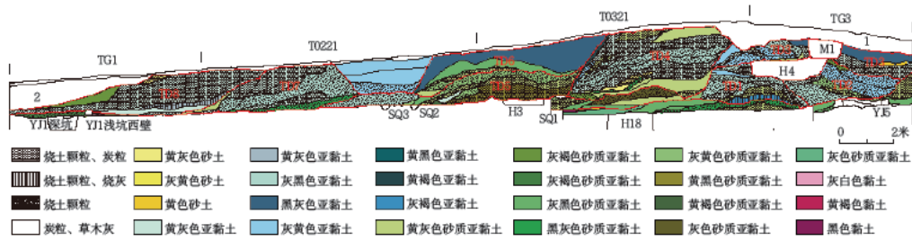
图四 发掘区南壁剖面图
