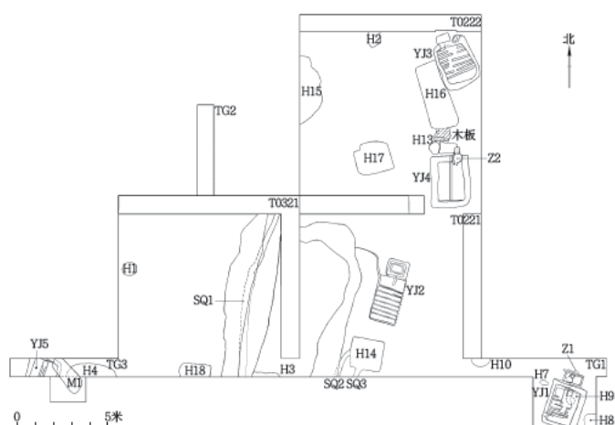
图二 发掘区平面图
