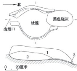
图一〇 Z2平、剖面图 1.灰黑色土 2.草木灰 3.黑色灰烬
