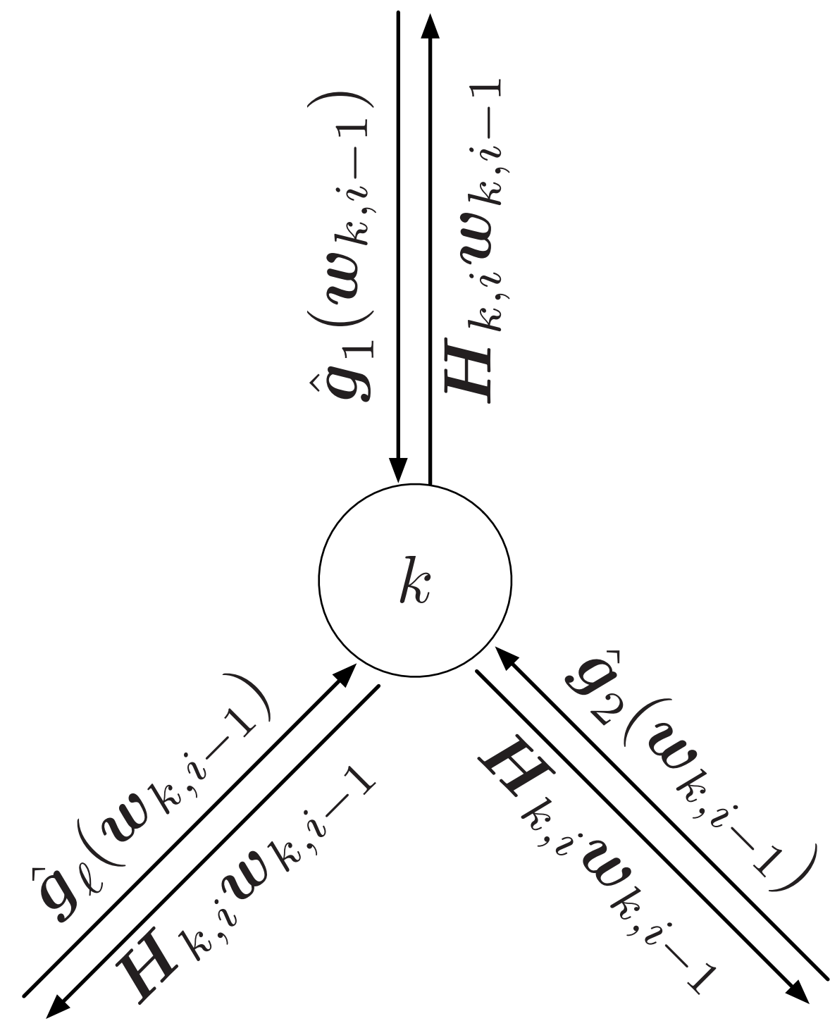
(d) Doubly compressed diffusion LMS
