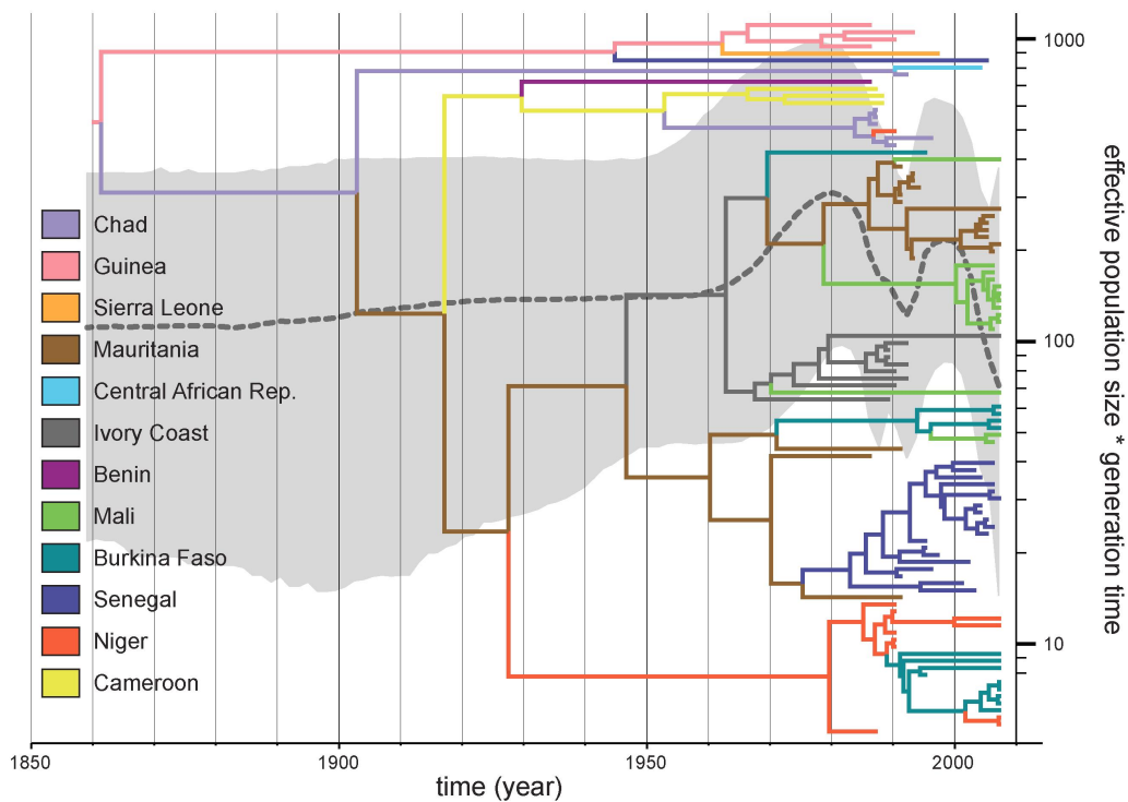
FIGURE 4 – Phylogéographie du virus de la rage en Afrique. Les couleurs de branches correspondent aux localisations ancestrales les plus probables du virus. En arrière-plan, la courbe en tirets et la zone grisée représentent la médiane et l'intervalle de crédibilité à 95 % de la taille de population effective. Cette figure correspond à la Figure 6A de [45].
