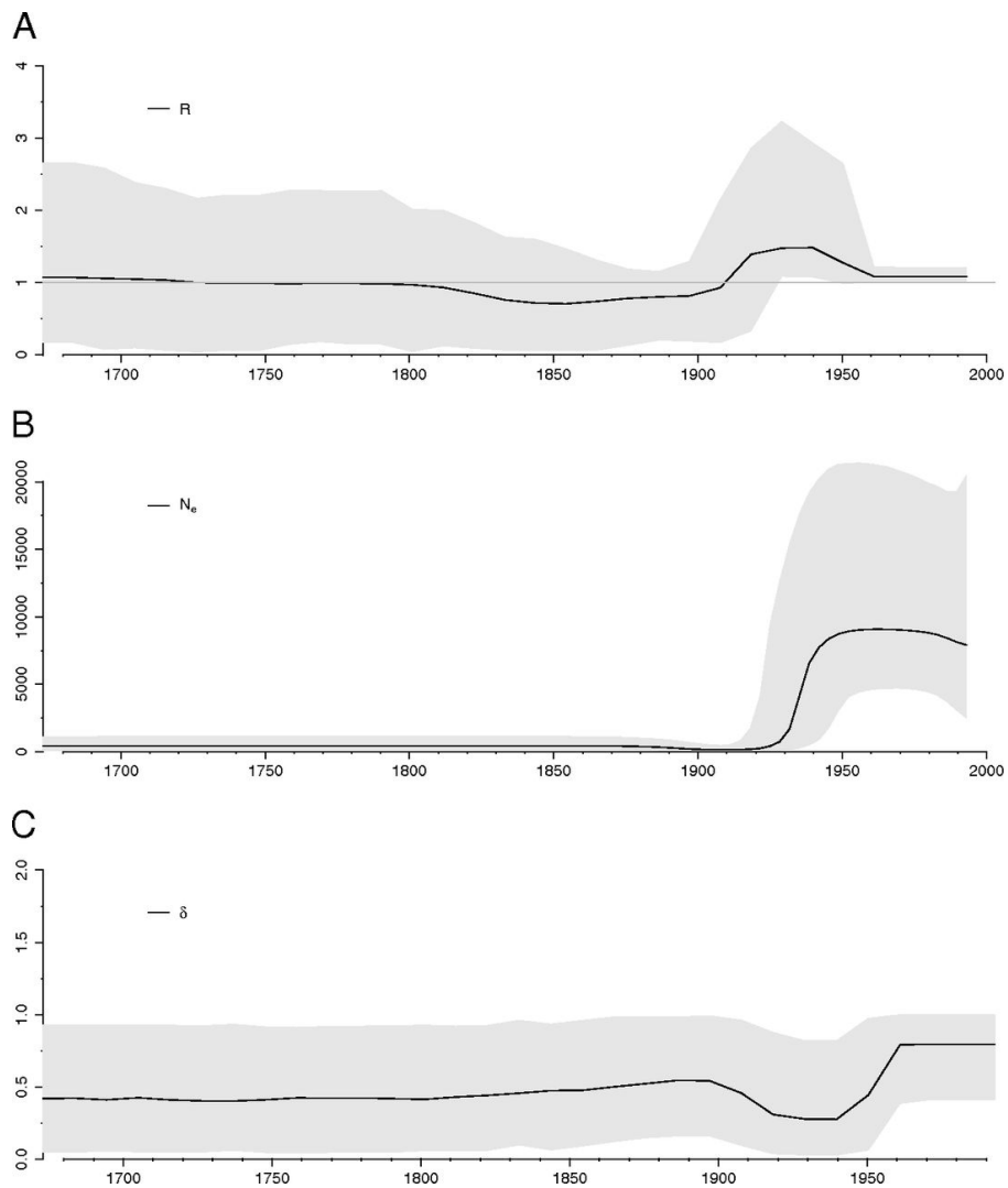
FIGURE 2 – Inférence phylodynamique bayésienne de l'épidémie de VHC en Égypte. A) Variation du taux de reproduction de base ( R_0 ), B) variations de la taille de population efficace ( N_E ) et C) variations du taux de fin des infections ( \delta ). Les lignes noires représentent les valeurs médianes inférées et les régions grisées les intervalles de crédibilité à 95 %. Cette figure correspond à la Figure 3 de [36].
