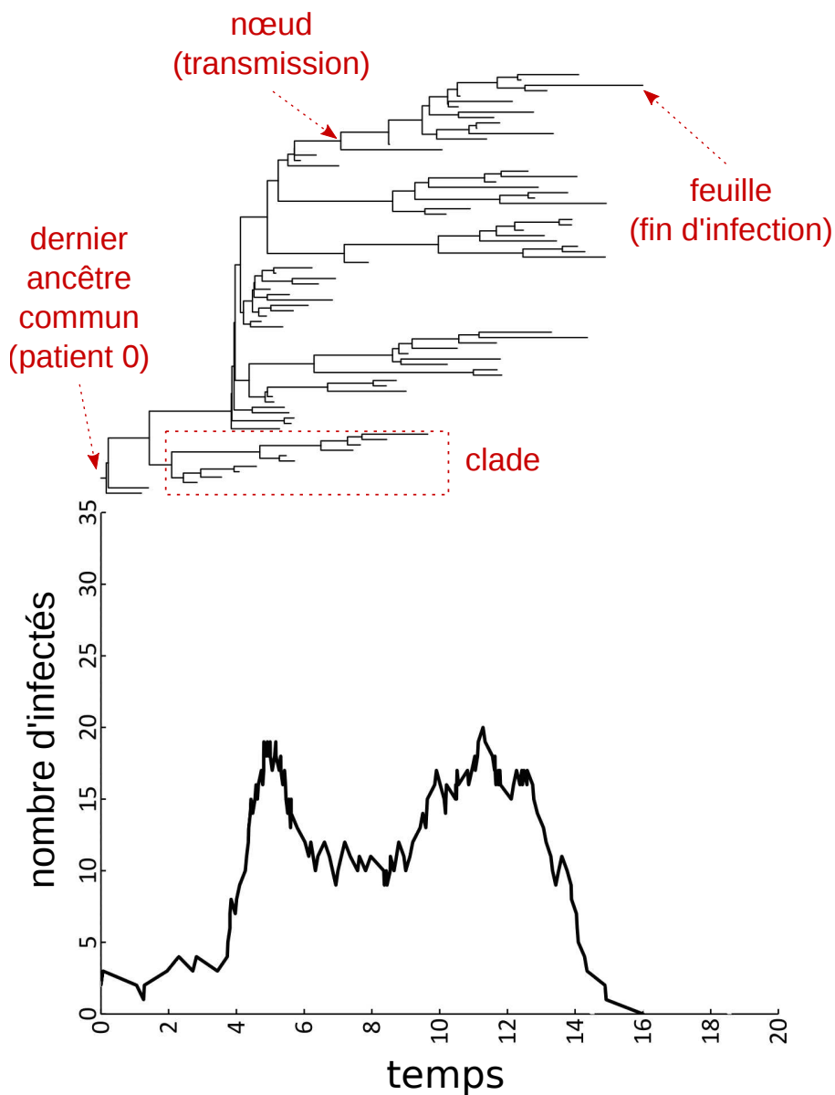
FIGURE 1 – Phylogénies correspondant à une épidémie. En haut, les éléments clés de la phylogénie sont décrits en rouge (voire aussi le Glossaire) et en bas une représentation « classique » d'une épidémie par une série temporelle de prévalence . On voit par exemple que l'augmentation du nombre de cas à partir de la 4 e unité de temps s'accompagne d'un foisonnement de branches dans la phylogénies. À l'inverse, la fin de l'épidémie se traduit par une abondance de feuilles dans la phylogénie. Cette illustration a été créée par Samuel Alizon et est mise à disposition sous une licence CC-BY 4.0.
