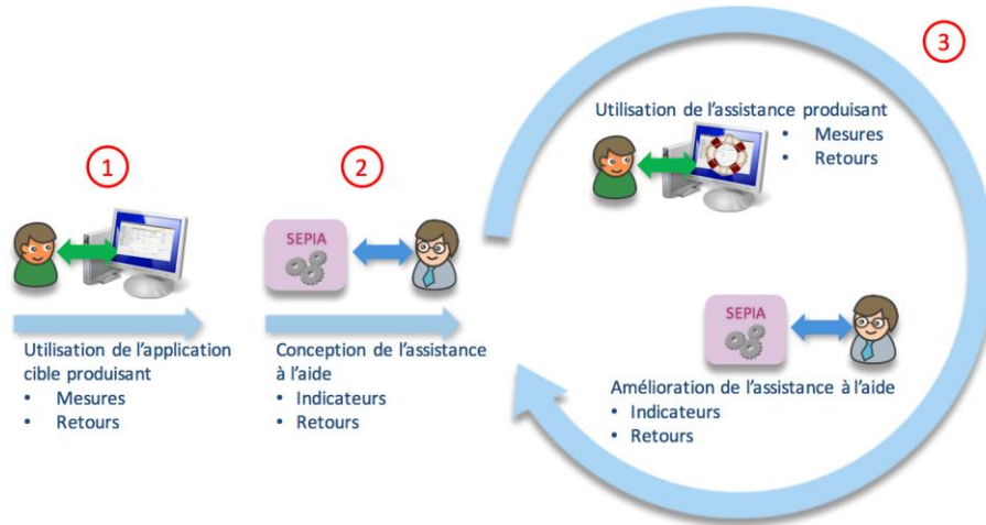
Fig. 3. Cycle de vie des systèmes d'assistance de SEPIA
