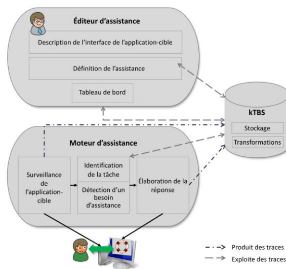
Fig. 2. Architecture du système SEPIA associé au kTBS.
