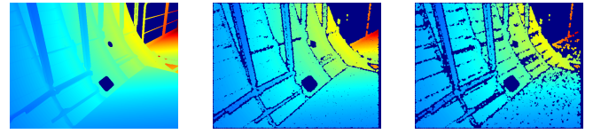
(a) Image de profondeur synthétique (b) Image de profondeur bruitée (modèle partiel) (c) Image de profondeur bruitée (modèle complet)
