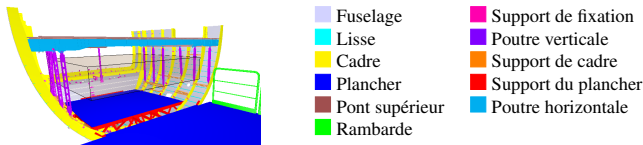
FIGURE 1 – Le maillage est représentatif d'un atelier d'assemblage sur lequel des robots assistants pourraient être déployés. La scène est divisée en 11 classes \mathcal{C} = \{c_1, \dots, c_{11}\} décrivant les structures de l'avion et une classe void en noir dans les exemples.
