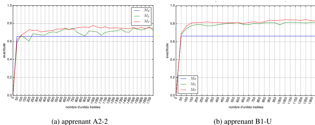
FIGURE 2: L'évolution incrémentale de la performance de M_P par rapport à M_L et M_E (50 unités lexicales/mini-lot). Nous présentons les limites inférieure (A2-2) et supérieure (B1-U) de performance.
