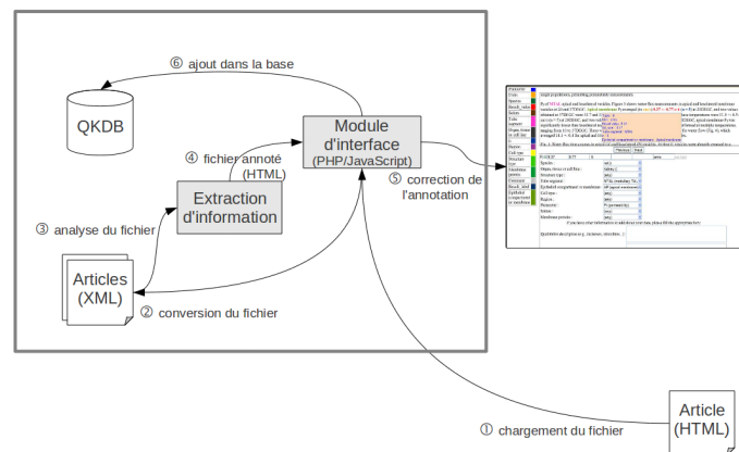
Figure 8. Architecture de l'assistant d'aide au peuplement de la base de données
