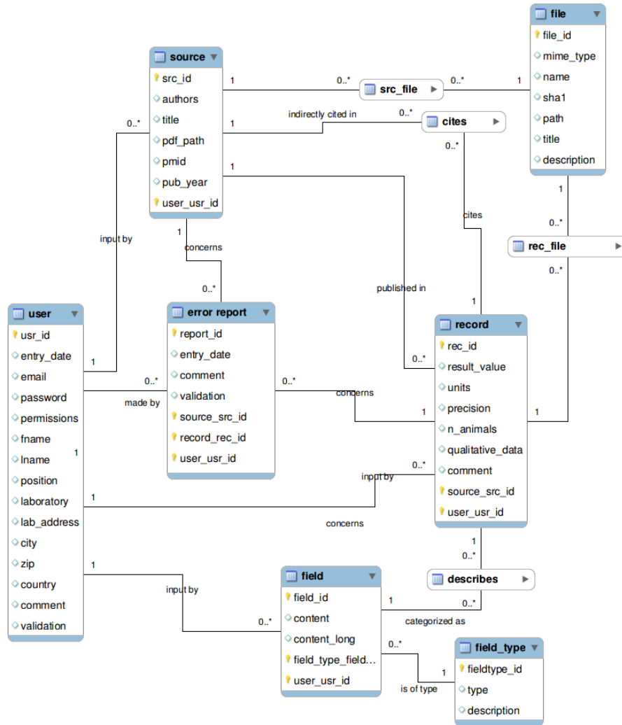
Figure 12. Schéma complet de la base de données QKDB
