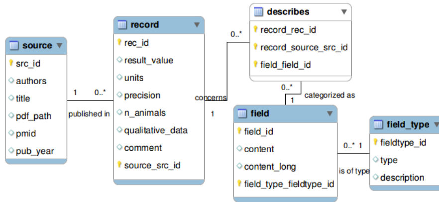
Figure 2. Schéma UML simplifié de la base de données QKDB
