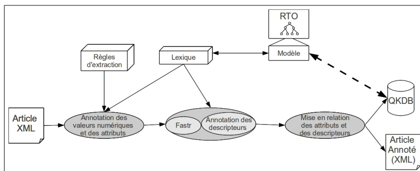
Figure 3. Schéma de fonctionnement du système d'extraction
