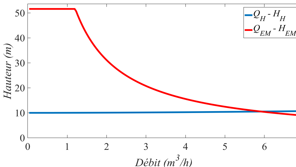
Figure 5 : Point de fonctionnement du système.
