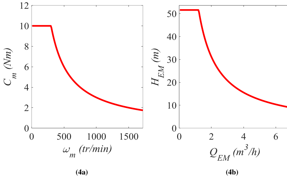
Figure 4 : (a) Couple sur l'arbre C_m en fonction de la vitesse de l'arbre \omega_m pour le moteur solaire (b) Hauteur générée par le système de pompage H_{EM} en fonction du débit délivré Q_{EM} .
