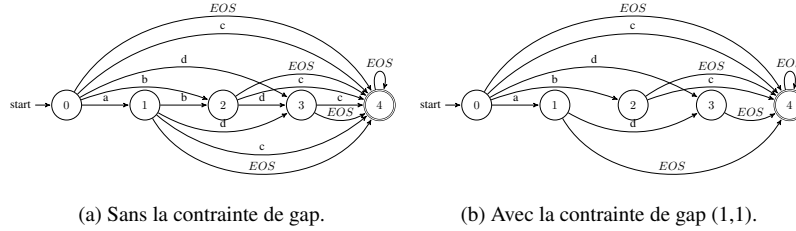
FIG. 1: Exemple d'automate pour la séquence \langle a b d c \rangle .
