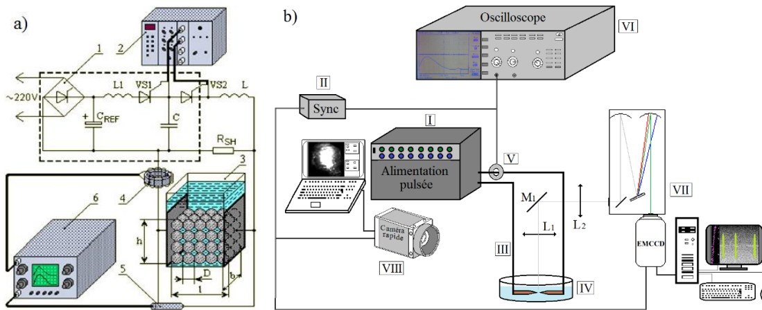
Figure 1. Dispositif expérimental (a) dispositif 1 à Kiev ; (b) dispositif 2 à Toulouse (la description détaillées des éléments de chaque dispositifs et donnée dans la section 2)
