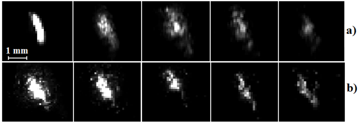
Figure 3. Photographies de la décharge obtenues par imagerie rapide (100 000 images/s), U \sim 100 V, I = 560 A, surface des électrodes sous 5 mm d'eau. (a) filtre à 780 nm, (b) filtre à 510 nm.
