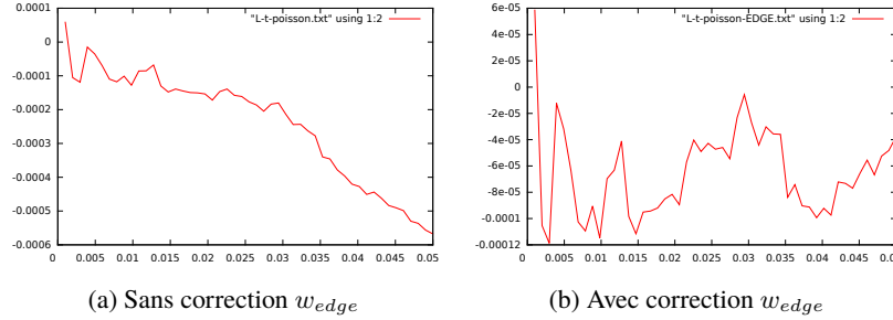
FIGURE 4 – Impact de la pondération sur \hat{L}(t) - t
