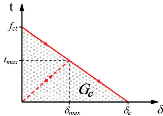
FIGURE 6 – Loi cohésive proposée par [34] (source [15])
