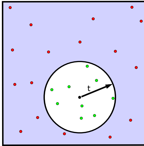
FIGURE 2 – Principe de la fonction K(t)
