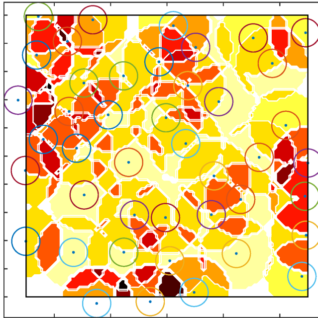
FIGURE 5 – Carte de clustering pour une répartition aléatoire
