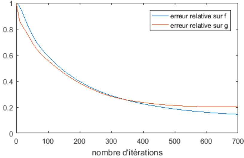
FIGURE 5 – Évolution de l'erreur relative sur le gain (en rouge) et le fond (en bleu) en fonction du nombre d'itérations.
