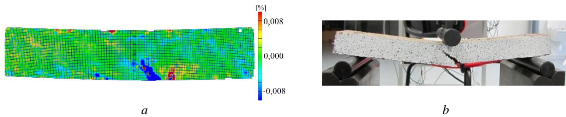
Figure 7 : Déformation \gamma_{zy} à une flèche de 4,7 mm (a) et rupture (b) d'une éprouvette B1_40 en flexion 3 points.
