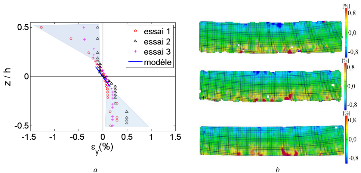
Figure 6: Evolution et variabilité de \epsilon_y d'une éprouvette B1_40 en flexion 3 points dans l'épaisseur totale (a) et champs de déformations des trois essais (b) pour une flèche de 2,5 mm.
