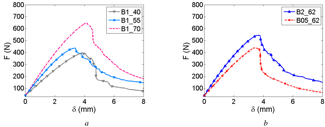
Figure 5 : Influence du taux de fibres (a) et du diamètre de fibres (b) sur l'évolution de la force en fonction du déplacement en flexion 3 points.
