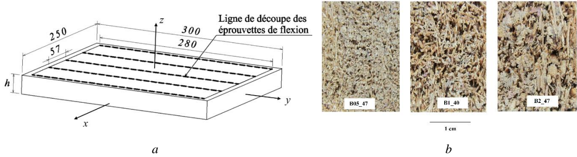
Figure 2 : Géométrie des plaques composites moulées et contour des éprouvettes de flexion. Notations et repérage. Unités en mm (a). Découpe dans le plan (yz) des matériaux B05_47, B1_40 et B2_47 (b).
