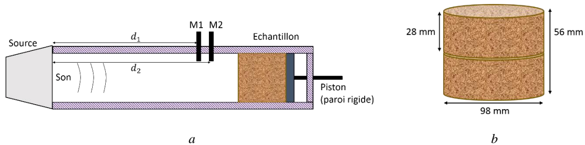
Figure 3 : Dispositif de mesure des pressions acoustiques dans un tube à impédance (a). Vue de l'échantillon d'épaisseur doublée (b).
