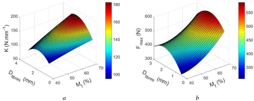
Figure 8 : Surfaces de réponses des propriétés issues de flexion 3 points en fonction du diamètre et du taux de fibres : K (a) et F_{max} (b).
