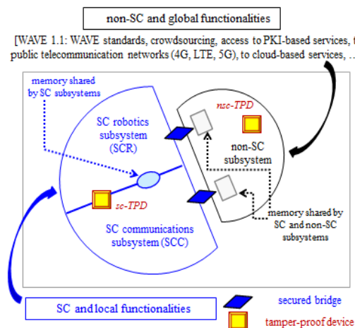
Figure 1. Exemple d'architecture d'un système bord
