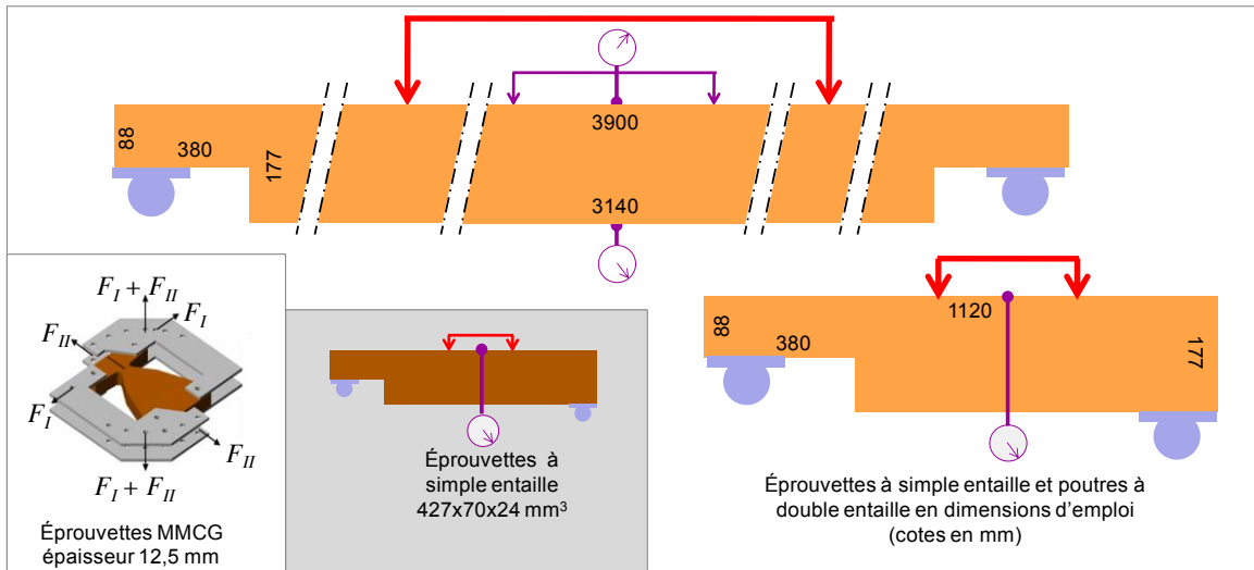
Figure 1. Types d'éprouvettes et poutres testées et échelles de ces corps d'épreuve
