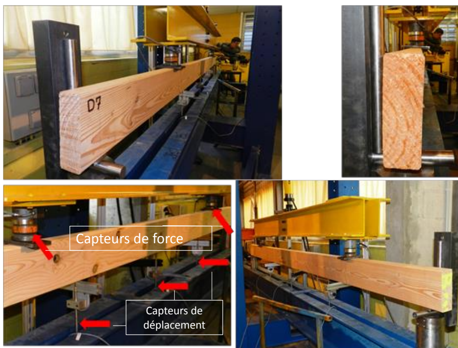
Figure 4. Configuration d'essais pour les essais de flexion quatre points sur poutres avant entaille.
