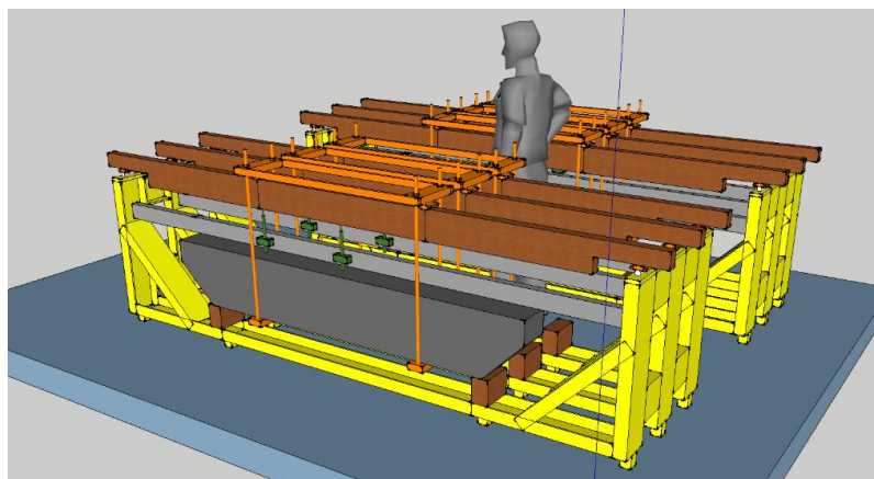
Figure 6. Configuration du bâti extérieur avec son système de chargement et son système de mesure.
