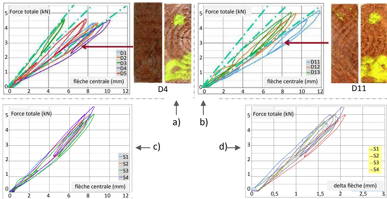
Figure 5. Comportement global d'une partie des poutres en Douglas et jumelage pour les poutres D4-D11.
