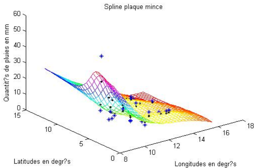
Figure 6. Spline Plaques Mince d'ajustement : Méthode multidimensionnelle avec tout le vecteur minimal
