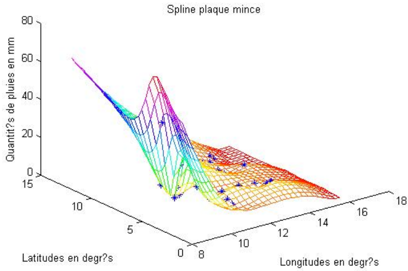
Figure 3. Splines Plaques Minces d'interpolation ( \rho = 0 ) sur les moyennes de pluies mensuelles
