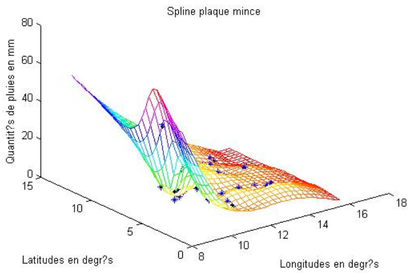
Figure 4. Spline Plaques Mince d'ajustement : Méthode heuristique avec la norme 2
