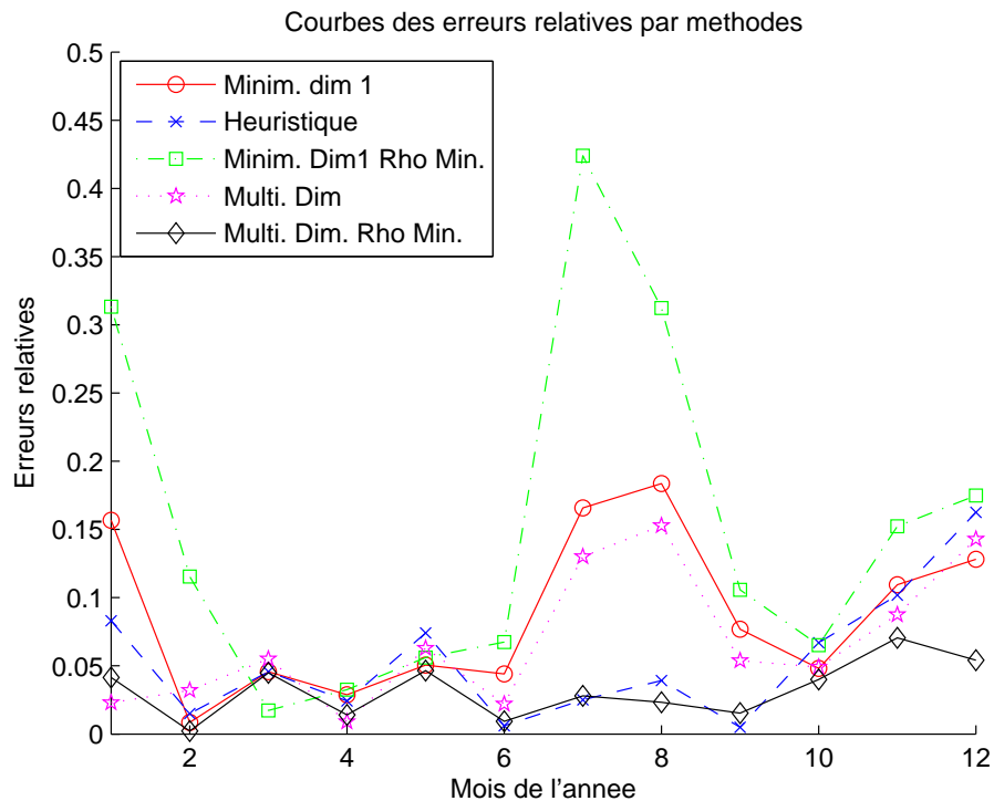
Figure 8. Courbe comparative des erreurs relatives sur les moyennes mensuelles au point de coordonnées L=13.11 \lambda=3.46
