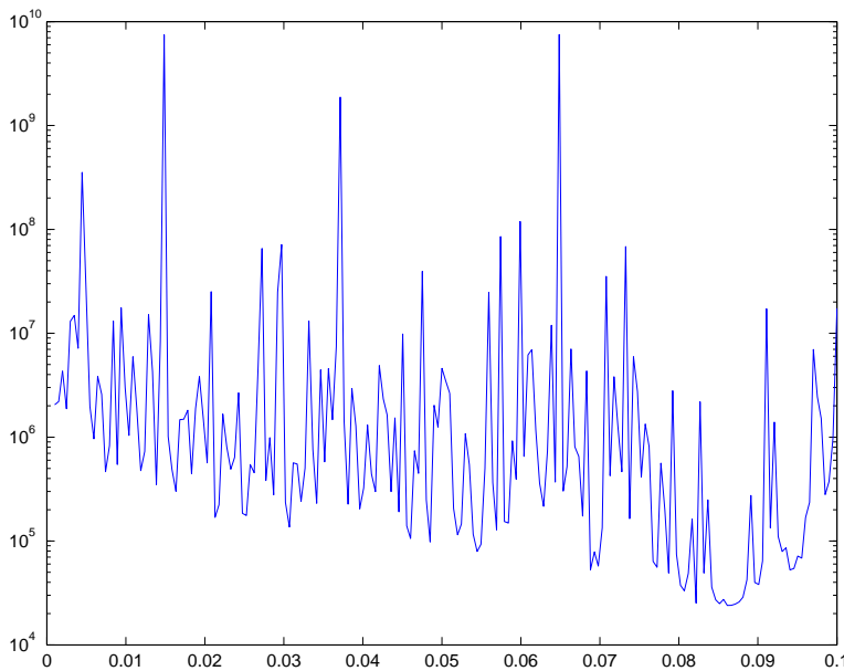
Figure 2. Courbe de V(\rho) pour la minimisation d'une variable
