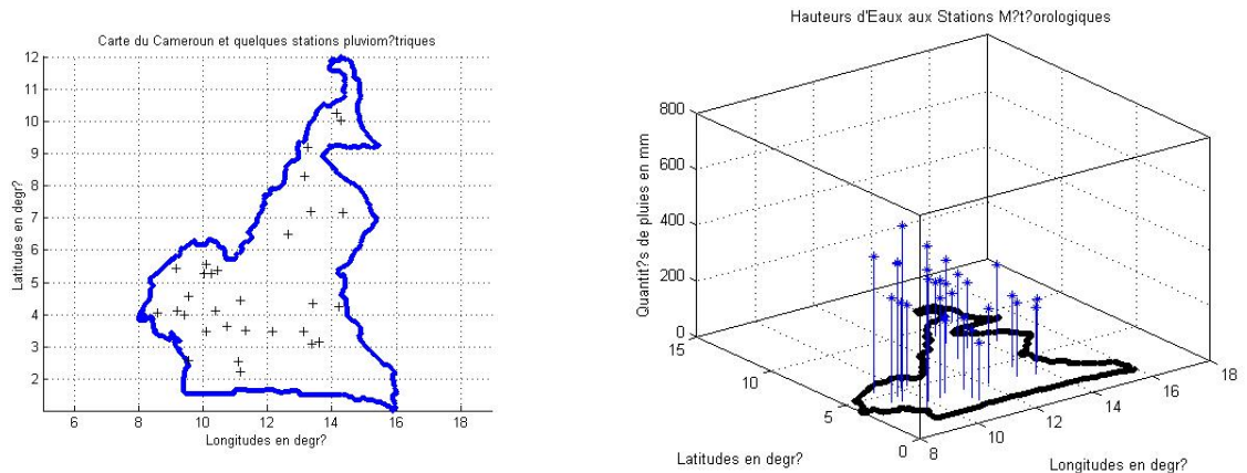
Figure 1. Stations et Hauteurs moyennes des pluies
