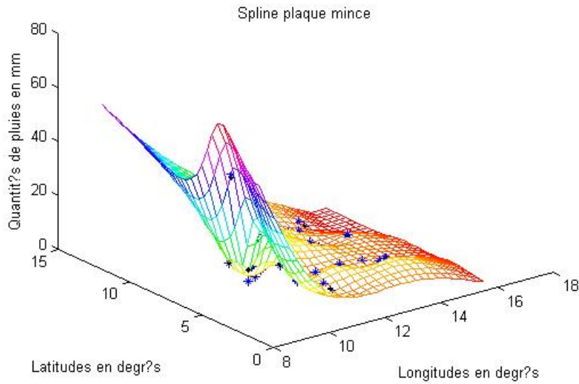
Figure 5. Spline Plaques Mince d'ajustement :Méthode multidimensionnelle avec le minimum du vecteur minimal sur les moyennes de pluies
