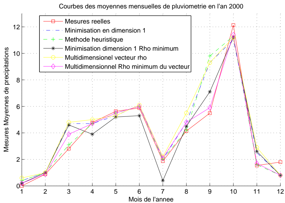
Figure 7. Courbe comparative des moyennes mensuelles au point de coordonnées L=13.11 l=3.46 Il ressort de la courbe 8 des erreurs relatives que la spline plaque mince d'ajustement construite par la méthode multidimensionnelle avec le minimum du vecteur minimal sur les moyennes de pluies, figure 5 et la spline plaques minces d'ajustement construite par la méthode heuristique avec la norme 2 sur la moyenne des pluies, figure 4 sont plus robustes. Pour ces deux splines les erreurs relatives sont de l'ordre de 10^{-2} , ordre de précision accepté à la Direction de la Météorologie du Cameroun.
