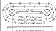
Fig. 3. — Schéma de l'installation des différents plans-mobles.
