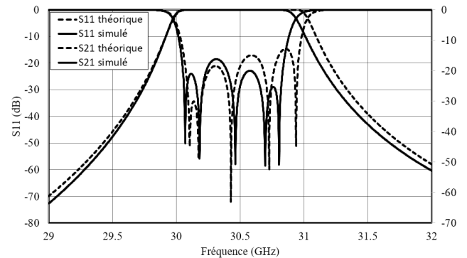
Fig. 7. Paramètres S du filtre en technologie SIW creux obtenus par simulation et du filtre obtenus par le calcul théorique.
