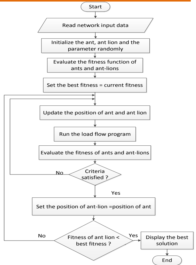
Fig. 5 Antlion optimizer.
