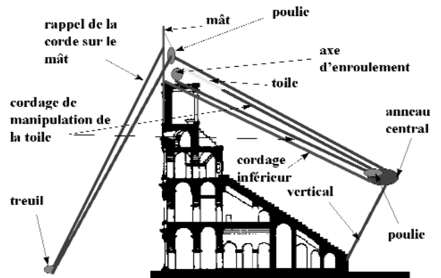
Fig. 6 : Plan des cordages du velum.
