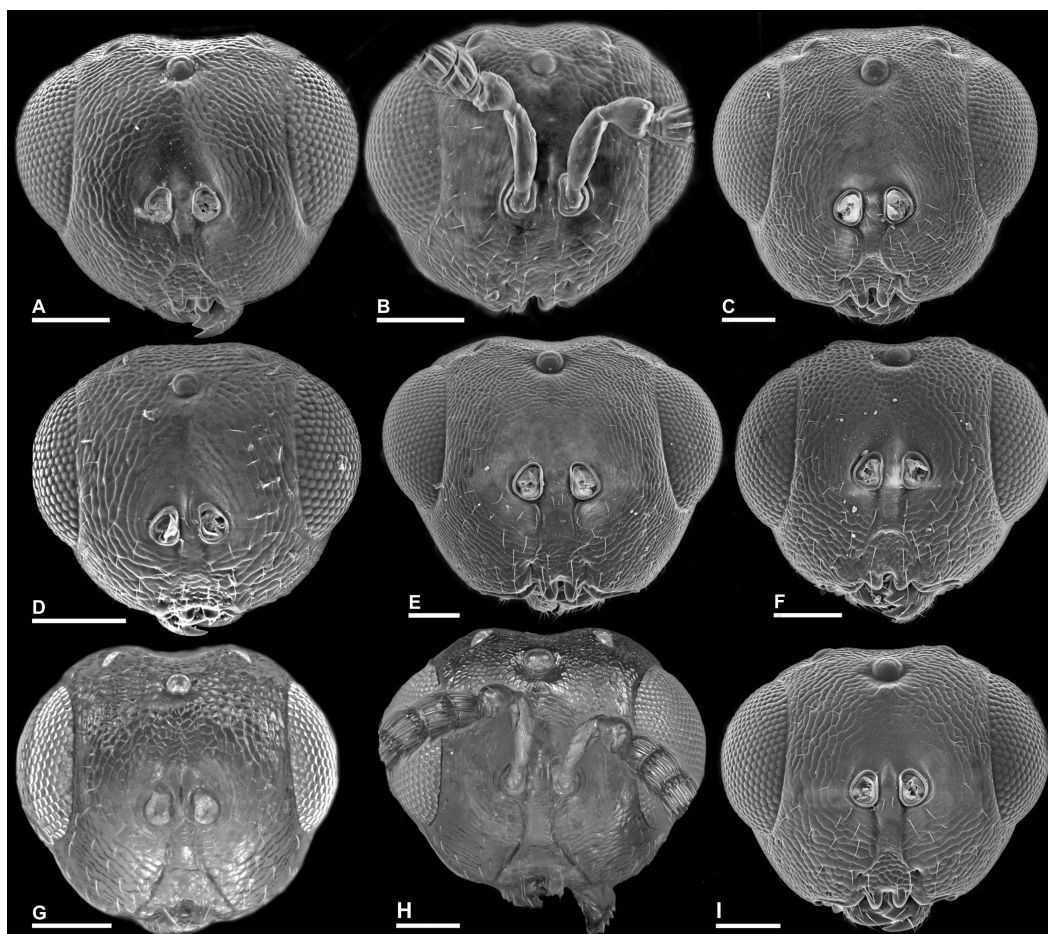
Figure 4 Head in frontal view, Idarnes incertus sp. group, females. (A) I. amacayacuensis sp. n.; (B) I. amazonicus sp. n.; (C) I. americanae sp. n.; (D) I. badiovertex sp. n.; (E) I. brevis sp. n.; (F) I. brunneus sp. n.; (G) I. comptoni sp. n.; (H) I. cremersiae sp. n.; (I) I. dimorphicus sp. n. Scale = 100 \mu m.
