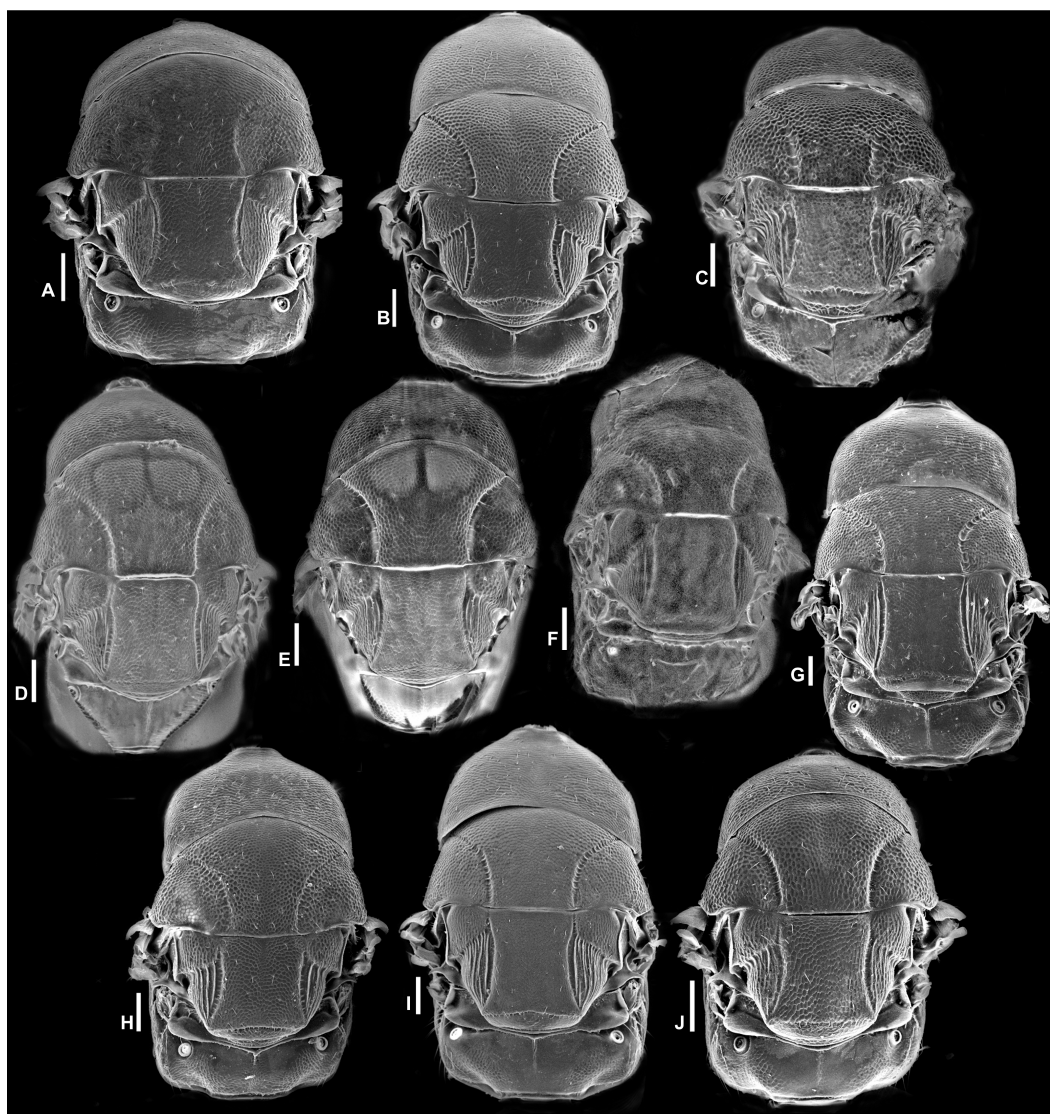
Figure 13 Mesosoma in dorsal view (SEM), Idarnes incertus sp. group, females. (A) I. flavicrus sp. n.; (B) I. flaviventris sp. n.; (C) I. gibberosus sp. n.; (D) I. gordhi sp. n.; (E) I. hansonii Bouček, 1993, Paratype; (F) I. incertus (Ashmead, 1900), Paralectotype USNM; (G) I. maximus sp. n.; (H) I. nigriventris sp. n.; (I) I. pseudoflavus sp. n.; (J) I. ramirezi sp. n. Scale = 100 \mu m.
