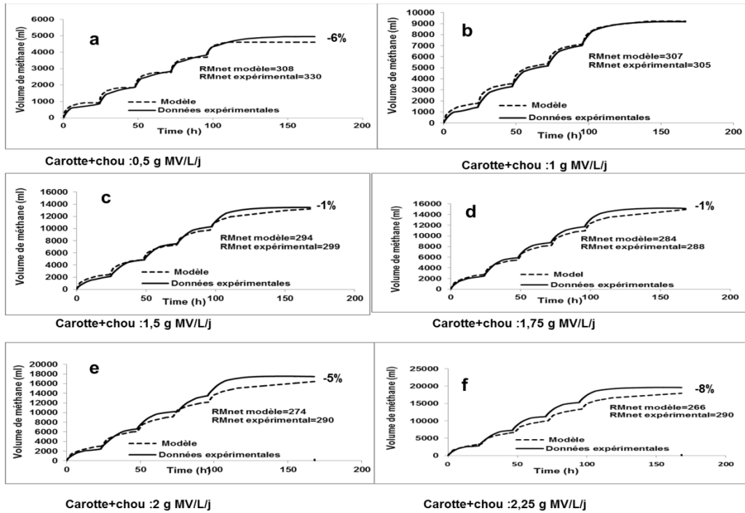
Fig. 1 : Comparaison entre les données expérimentales nettes et les données modélisées pour le mélange carotte + chou à des charges appliquées croissantes.
