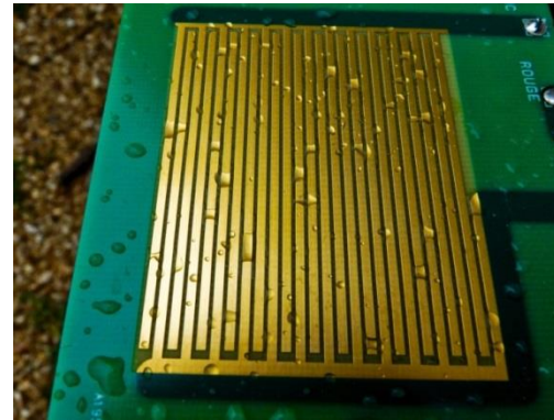
Capteur Campbell 237
