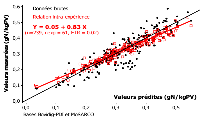
Figure 3 : Evaluation de la prédiction des rejets azotés urinaires par les vaches laitiers
