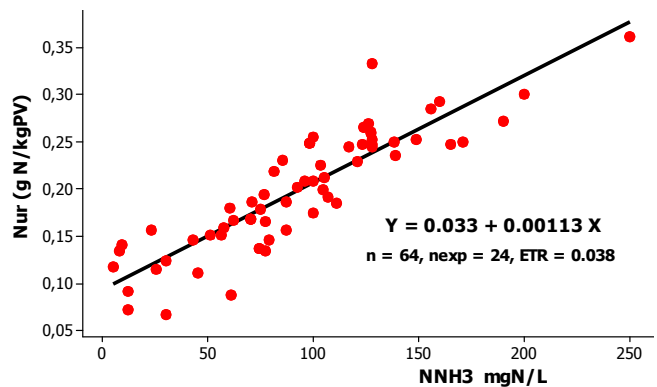
Figure 2 : Influence de la teneur en N-NH3 du jus de rumen sur les rejets Nur chez les bovins (Base Bovidig).
