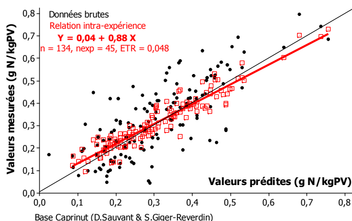
Figure 4: Evaluation de la prédiction des rejets azotés urinaires par les chèvres laitiers
