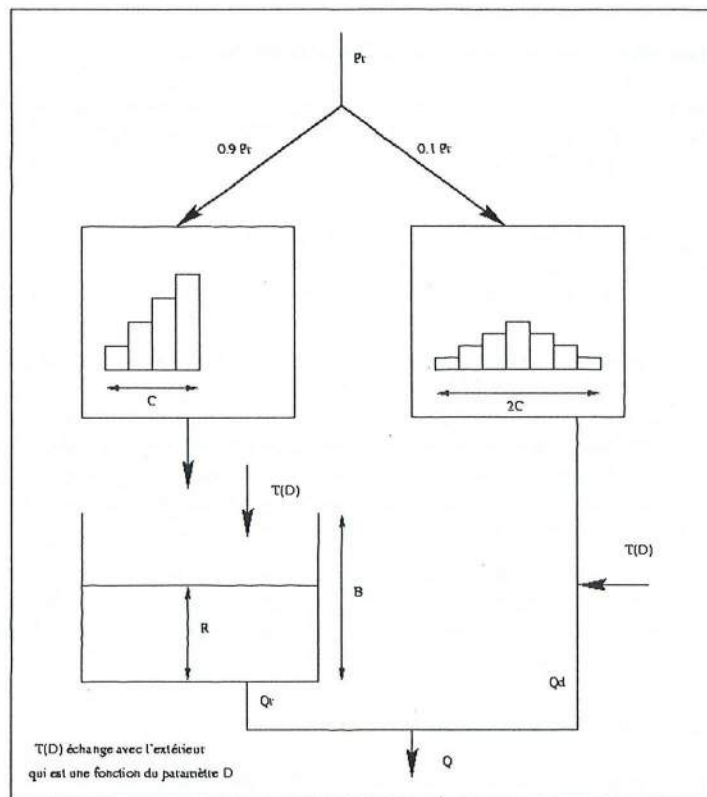
Figure 2 Représentation schématique de la fonction de transfert du modèle GR4
