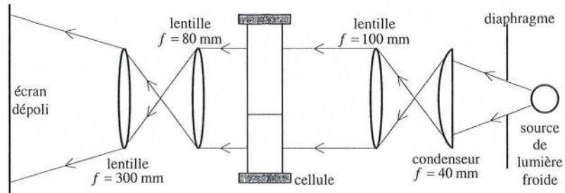
Figure 4 : schéma de principe de la méthode d'ombroscopie.
