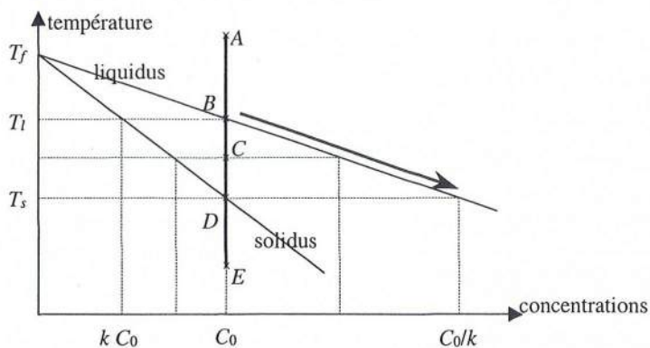
Figure 1 : diagramme d'équilibre binaire de l'eau et d'un sel faiblement concentré.
