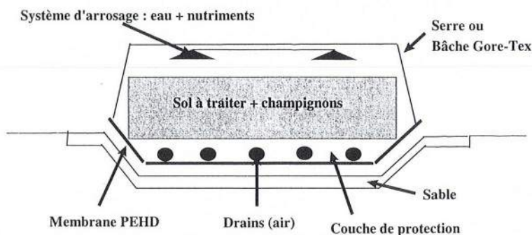
Figure 1 : Mise en œuvre du traitement de sol en biotierre
