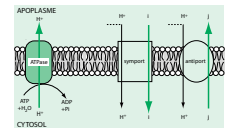
Figure 2.6 - Principe de fonctionnement des transports actifs secondaires de la membrane plasmique. Les ions sont transportés activement soit dans le sens de l'efflux (E) soit dans le sens de l'efflux (I). L'ATPase pompe à l'extérieur un gradient de \text{Na}^+ à travers la membrane. Le gradient est alors utilisé pour diriger un flux de \text{Na}^+ en retour vers le compartiment d'origine (le cytosol) à travers des systèmes de transport actifs (ou Au retour des températures de nos ions, la force de retour opératoire de \text{Na}^+ est opposée à l'entrée active de l'ion (symport), soit à la sortie active de l'ion (antiport).
