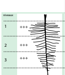
Figure 2.16 - Influence sur l'axe de la répartition des ions nitrate ( \text{NO}_3^- ) dans une racine végétale.
