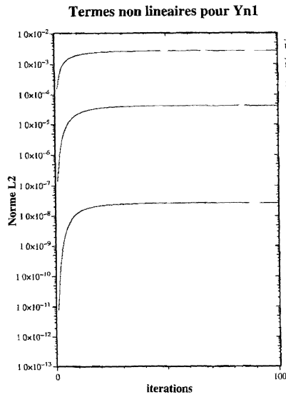
Figure 5. — Influence de la composante non linéaire sur les plus grandes structures.
