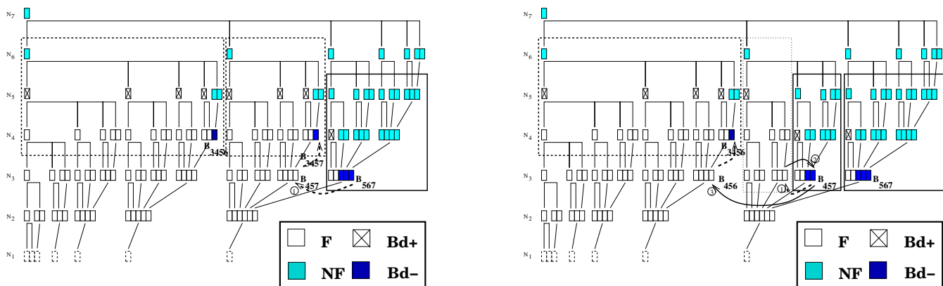
FIG. 7 – Changement de niveau (de k à k + 1 ). Ici \alpha = 3 , N = 7 . Le traitement est différent selon que la taille du bloc \mathcal{B}_Y qui aurait dû être traité au niveau k est \geq \alpha (à gauche) ou = \alpha (à droite).
