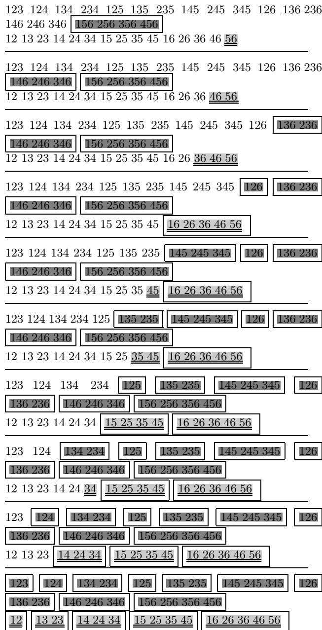
FIG. 3 – Légende : bordure négative , bordure positive . Évolution des bordures lors de la construction d'une bordure négative de distribution \langle \mathcal{B}d^- \rangle = \langle 0, 0, 20 \rangle selon [DDM05]. Seuls les niveaux utiles 2 et 3 sont présentés. De haut en bas apparaissent chacune des étapes amenant de nouveaux motifs dans \mathcal{B}d^+ . Cet exemple met en évidence que l'intégration d'un motif ou quelquefois plusieurs motifs dans la bordure positive correspond à l'intégration dans la bordure négative d'un « bloc » de sur-motifs consécutifs dans l'ordre colex. La solution apparaît dans le « pavé » du bas.
