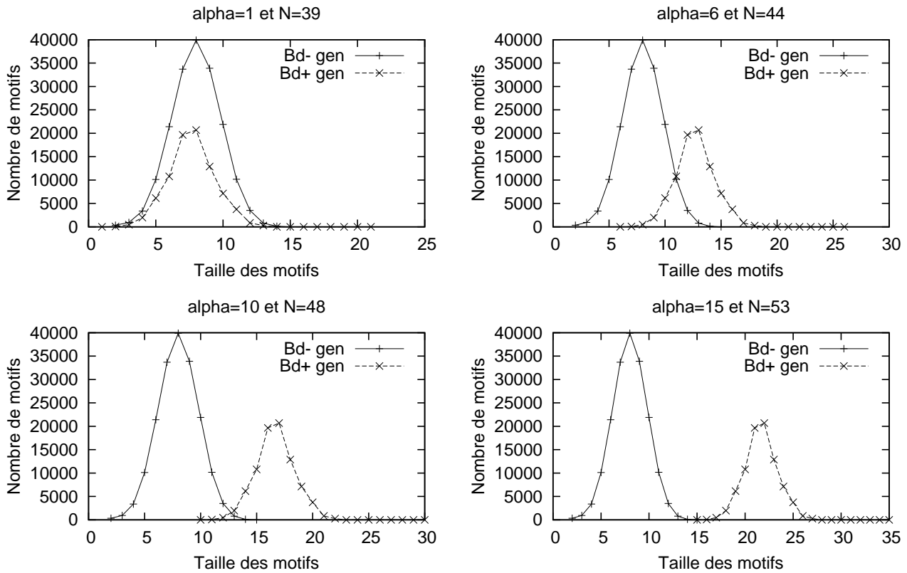
FIG. 9 – Influence de \alpha pour Chess 30% ( \alpha = d + 2 )
