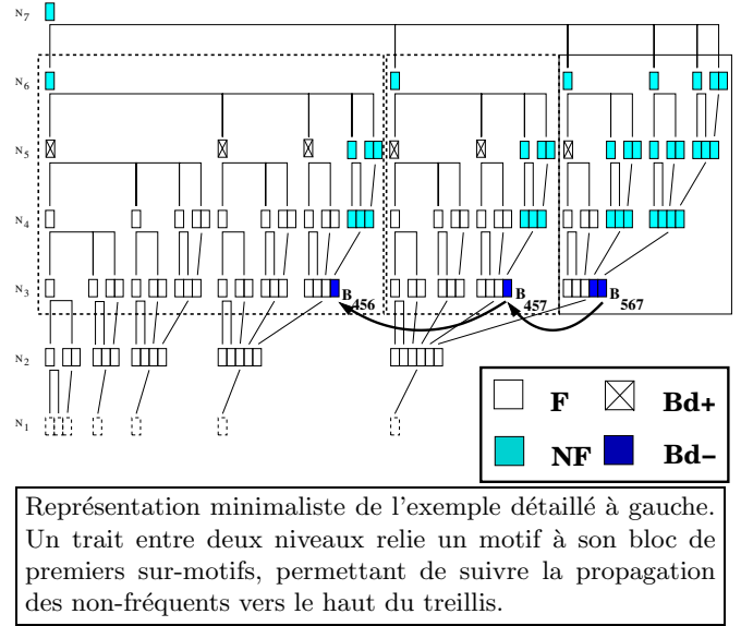
FIG. 4 – Exemple de construction d’une bordure négative sur un seul niveau avec un paramètre d’éloignement \alpha = 4 (algorithme 3 avec : \alpha = 4 , \mathcal{S}^- = \langle 0, 0, 4 \rangle , N = 7 ). Seuls les motifs de rang \geq 4 dans leur bloc sont intégrés. La bordure positive correspondante est éloignée de \alpha - 2 = 2 niveaux.
