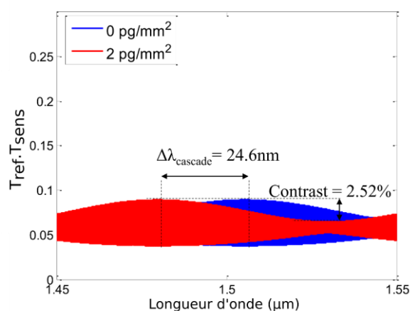
Fig. 2 : Spectre de transmission calculé d'un capteur à effet Vernier hybride
