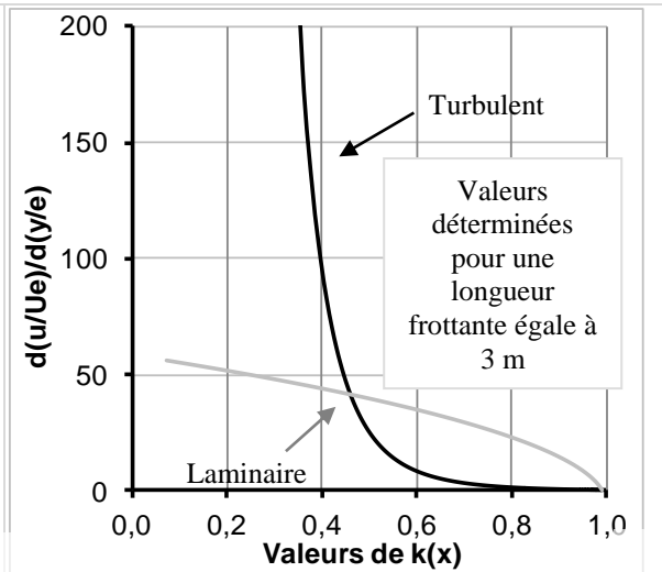
Fig.7 – Évolution des gradients des vitesses transversales rapportés à la vitesse infinie amont U_e et à l'épaisseur e du milieu poreux en fonction du rapport des vitesses k(x) pour v_o = 15 \times 10^{-6} \text{ m}^2/\text{s} .
