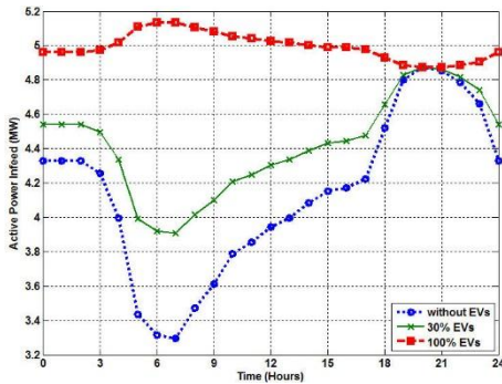
Fig. 29. Load profile of Fdr1
