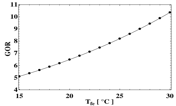
Figure 6 : Effet de T_{fe} sur le GOR
