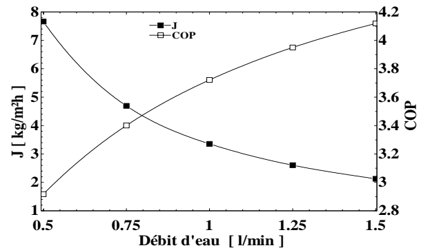
Figure 7 : Effet du débit sur le flux de perméat et le COP
