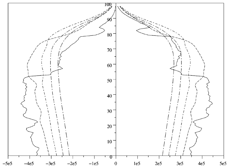
FIGURE 1 – Sans immigration. (a) Naissances totales : x \mapsto B_{1,2}(x) + B_{2,2}(x) . Mortalités : x \mapsto d_1(x) et x \mapsto d_2(x) . (b) À gauche : P_1(x, t) . À droite : P_2(x, t) . Ligne continue : situation en 1999. Lignes en pointillé : projections après 25, 50, 75 et 100 ans.
