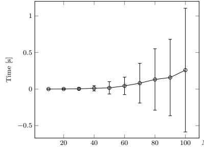
(d) Interpolation of average execution times of Table 16c.
