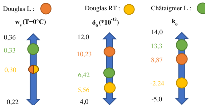
Figure 4: Valeurs de trois paramètres (teneur en eau de saturation, coefficient de perméabilité apparente (vapeur), coefficient de perméabilité apparente (eau adsorbée), selon l'essence et le sens de diffusion après identification)
