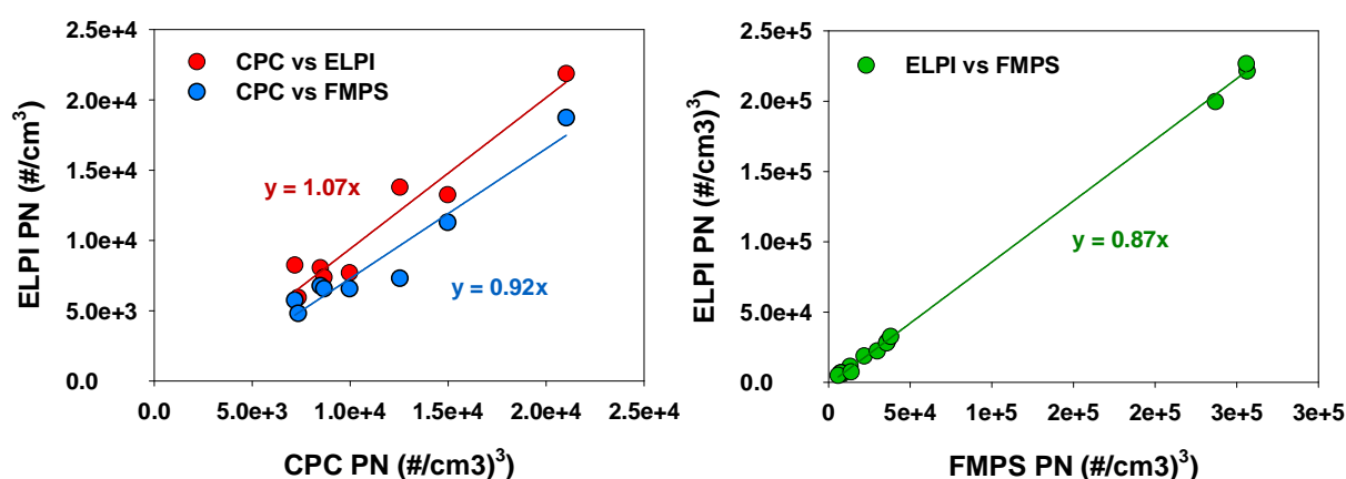
Figure 2. Comparaison des concentrations des particules mesurées par le CPC, l'ELPI et le FMPS pour l'ensemble des conditions expérimentales.
