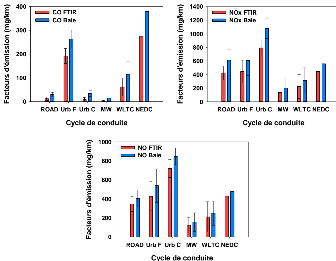
Figure 5. Comparaison entre les mesures du FTIR (bar rouge) et de la baie d'analyse (bar bleu) pour le CO, NO x et NO, avec les cycles Artémis Urbain, Routier, Autoroutier, WLTC et NEDC
