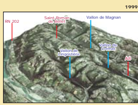
Vues "3D" des collines de Bellet en 1955 et 1999 : orthophotos drappées sur MNT 20 m
