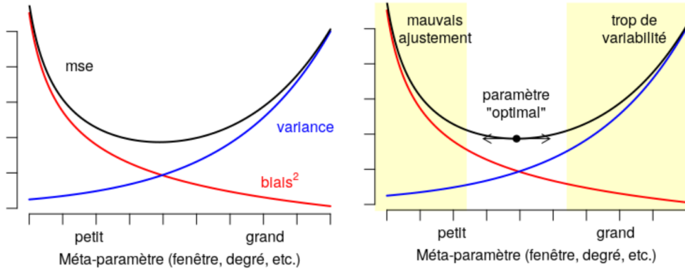
Figure 1: Choix de h et le problème de Boucle d'Or : h ne doit être ni trop grand (sinon il y a trop de variance), ni trop petit (sinon il y a trop de biais) .
