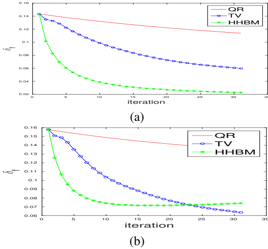
FIGURE 3 – Comparaison du NMSE du fantôme de Shepp Logan reconstruit de taille 64^3 en utilisant différentes méthodes avec 64 projections et SNR (a) 40dB et (b) 20dB.
