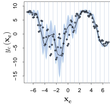
(d) 20 observations : A posteriori linearized
