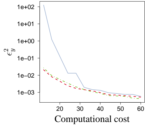
(d) Hydrodynamic example : Prediction
