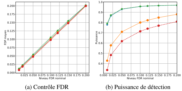
FIGURE 2 – (a) FDR empirique vs FDR nominal ; (b) : puissance vs FDR nominal. Méthode proposée : *, l'approche non-connexe : o. En trait plein, la détection est faite sur une fenêtre 51 \times 51 , en pointillés sur une zone 71 \times 71 (même cible de taille 360 pixels). Résultats moyennés sur 500 simulations Monte-Carlo.
