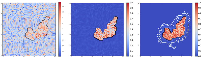
(a) Réalisation bruitée (b) Détection par méthode non-connexe (c) Détection par COMET
