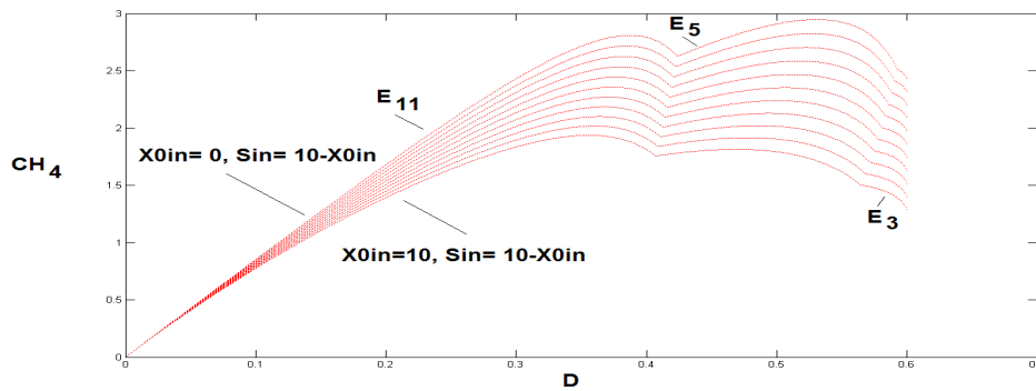
Figure 9. La variation du taux maximal du méthane pour S_{in} + X_{0in} = 10 , 0 \leq D \leq 0.6 , \mu_h = 1 , \mu_a = 5 et k_I = 10 .
