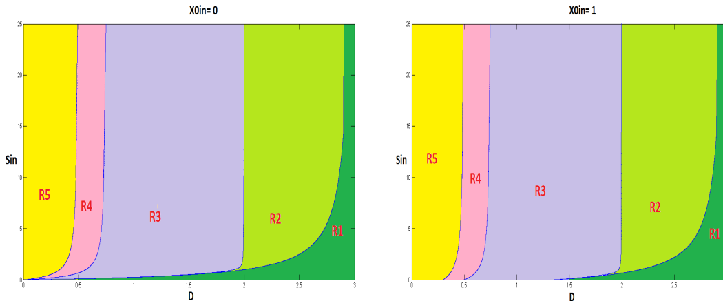
Figure 2. Diagramme opératoire, dans le plan (D, S_{in}) , à gauche pour X_{0in} = 0 , à droite pour X_{0in} = 1 .
